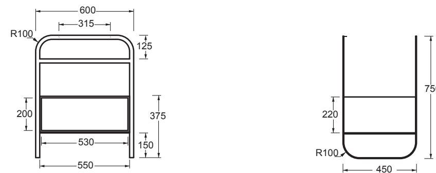
STRUTTURA CASSETTO structure with top per LUNARIS 81x45
