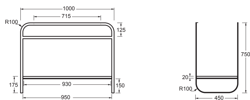
STRUTTURA PIANO structure with top per LUNARIS 121x45
