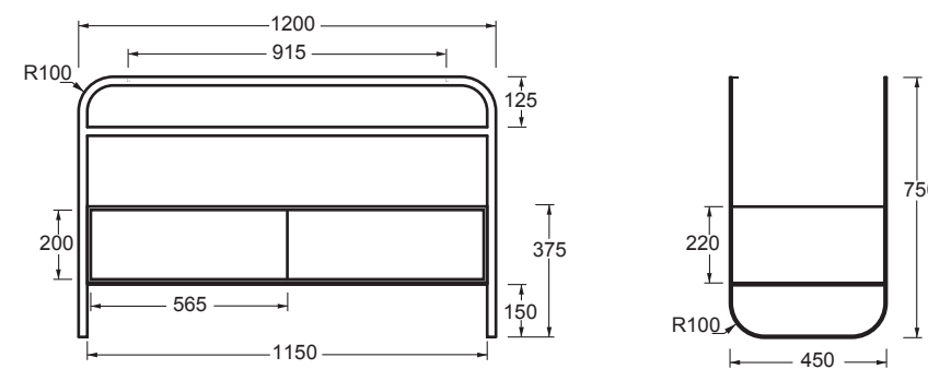
STRUTTURA CASSETTO structure with top per LUNARIS 121x45
