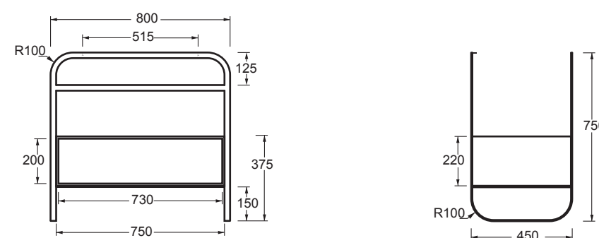
STRUTTURA CASSETTO structure with top per LUNARIS 101x45
