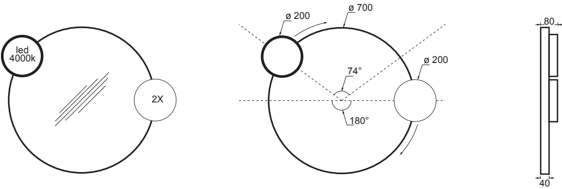
SPECCHIO Mirror ø70
