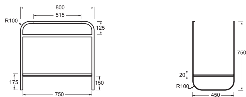
STRUTTURA PIANO structure with top per LUNARIS 101x45
