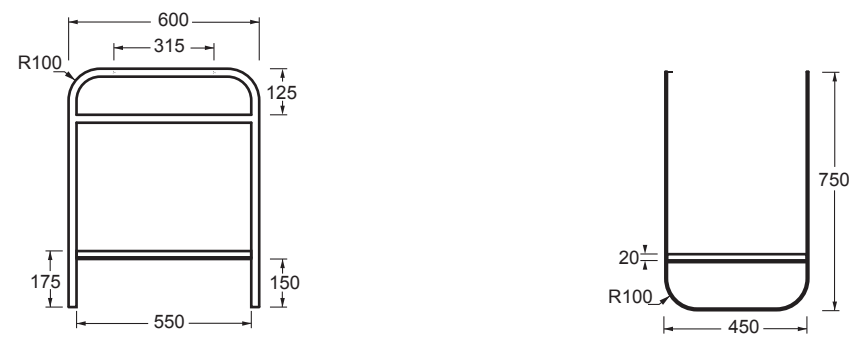
STRUTTURA PIANO structure with top per LUNARIS 81x45
