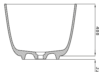
Sezione B-B
